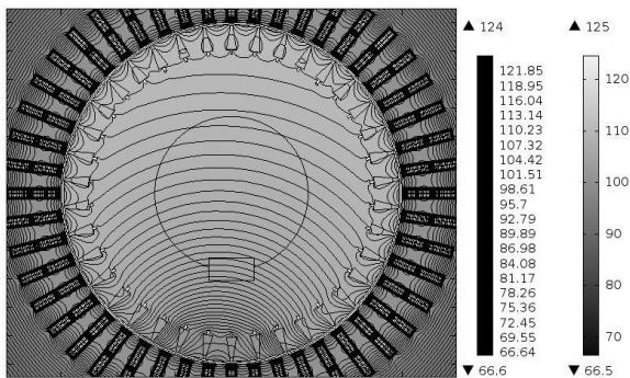
Рис. 5 – Температура в роторі АД при 5-ти uszkodжених сегментів КЗК
