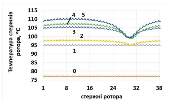
Рис. 6 – Температура в стержнях ротора в залежності від кількості uszkodжених сегментів КЗК
