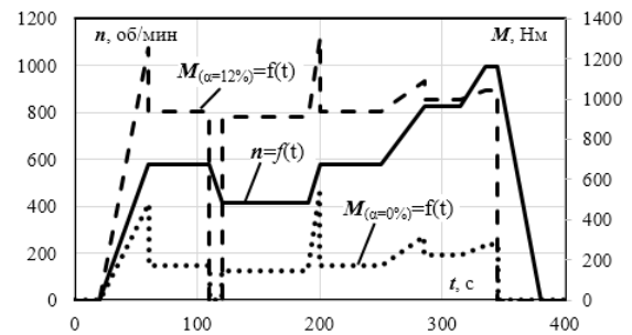
Рис. 2 – Зависимость момента, необходимого для движения автомобиля, и частоты вращения колес согласно загородному ездовому циклу
