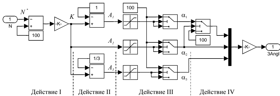
Рис. 4 – Структурная схема блока Angles
