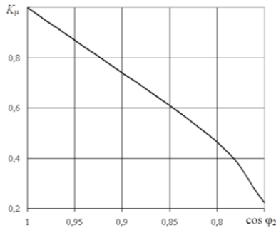
Рис. 5 – Графік залежності K_{\sigma} = f_2(\cos \varphi_2)
