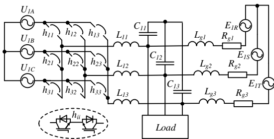
Рис.1 –Схема електрична
