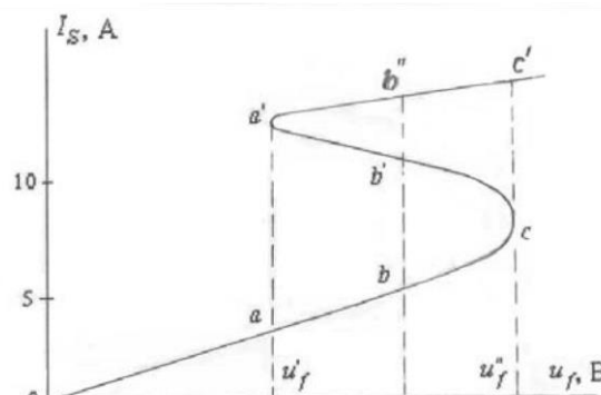
Рис. 3 – Залежність діючого значення струму якоря від напруги збудження модельного синхронного генератора, яка ілюструє багатозначність періодичних режимів при ферорезонансі
