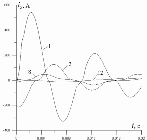
Рис. 6 – Розрахункові криві струму якоря на дванадцяти ітераціях, що призвели до нестійкого режиму модельного синхронного генератора
